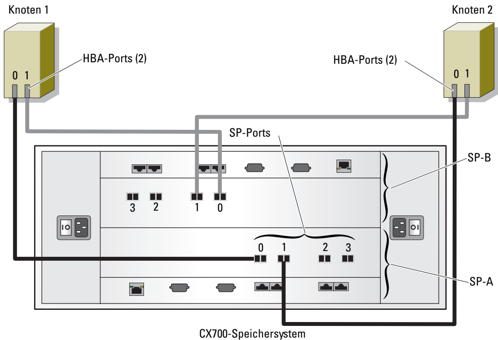
Abbildung 1-2. Fibre-Channel-Cluster mit Direktanschluss verkabeln
